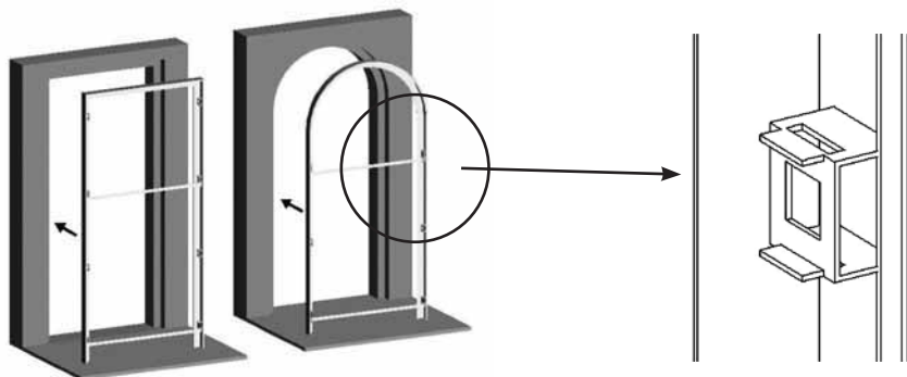
Particolare "gabbietta" di fissaggio del telaio al controteelaio
