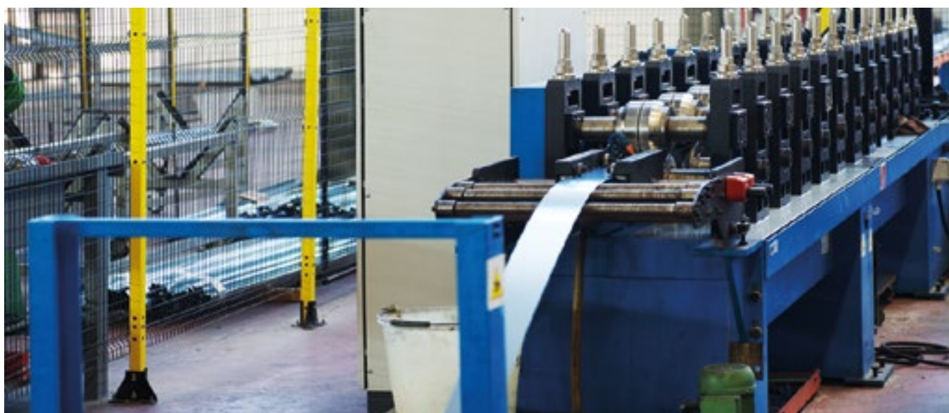
Profilatura lamiera per produzione strutture metalliche per porte. Profiling department for door metal trackset production.
