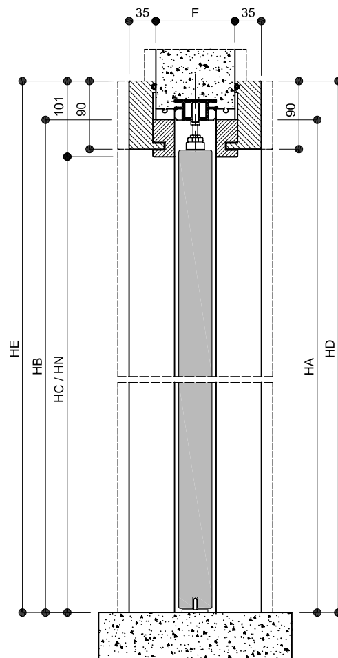
Sezione / Section B - B
