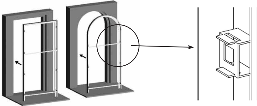
Particolare "gabbietta" di fissaggio del telaio al controte laio
