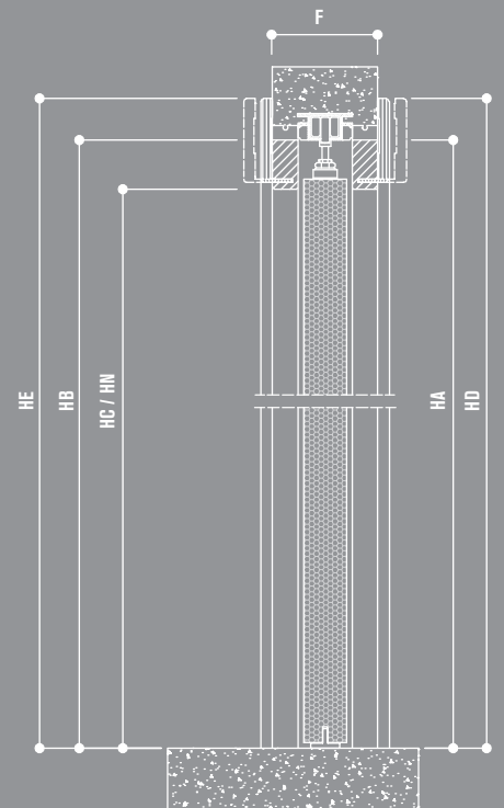
Porta Scorrevole interno muro / Hidden Sliding door
