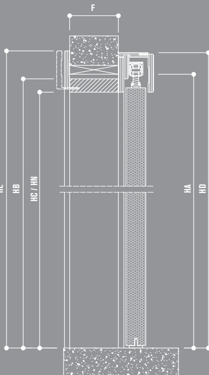
Porta Scorrevole esterno muro / Sliding door
