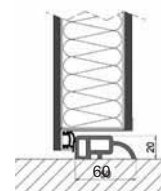
soglia con battuta singola
