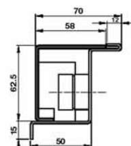
accoppiamento telaio e contro telaio
